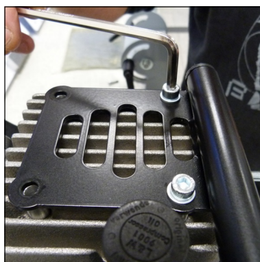
Abb. 3 - Ventilkopfschrauben lösen
