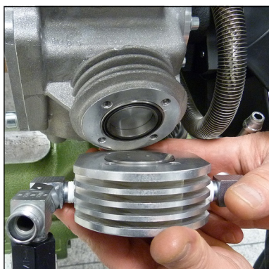
Abb. 3 - Ventilkopf mit Saug- und Druckventil entnehmen
