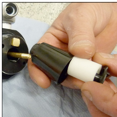
Abb. 5 - Sinterfilter wechseln
