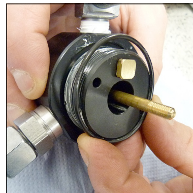
Abb. 6 - O-Ring wechseln
