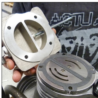
Abb. 7 - Ein- und Auslasskanäle müssen genau zentriert sein
