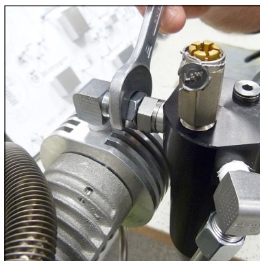
Abb. 2- Rohrleitungsverschraubungen lösen
