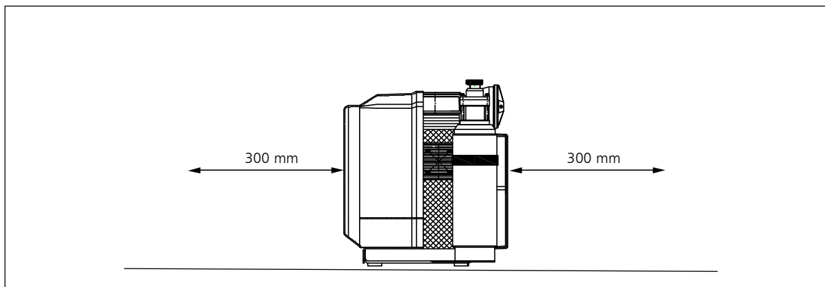
Abb. Mindestabstände LW 100 B
