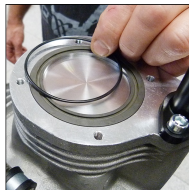
Abb. 5 - O-Ring wechseln
