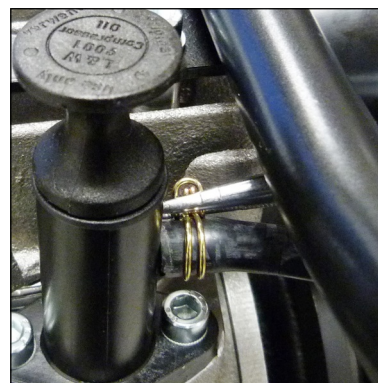
Abb. 9 - Klemmring befestigen
