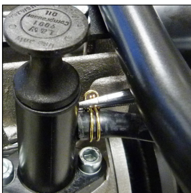
Abb. 2 - Klemmring entfernen
