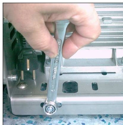
Abb. 2 - Spannmutter Antriebsmotor
