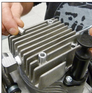
Abb. 8 - Distanzröhrchen aufsetzen
