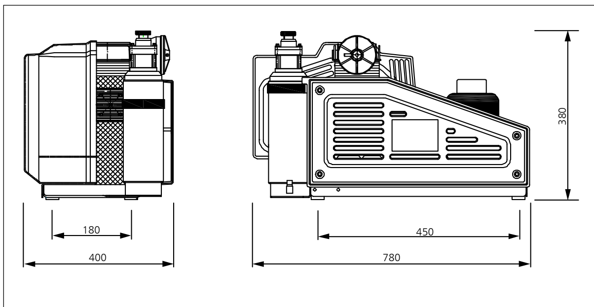
Abb. Einbaumaße
